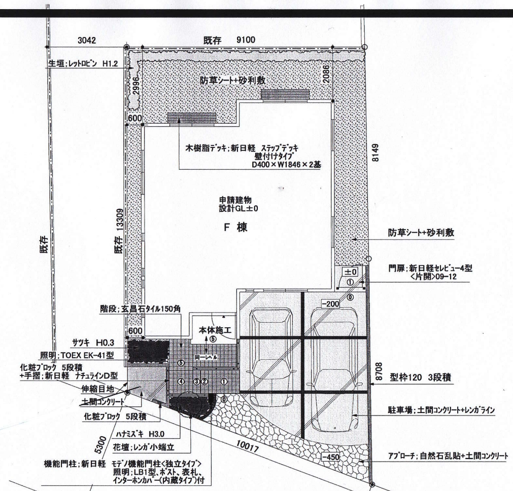
平面図 S=1/100
