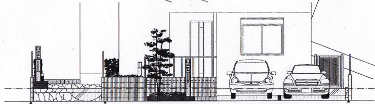
立面図 S=1/100
